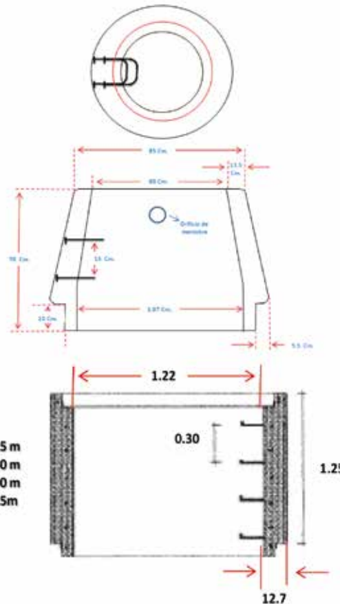
■ LÍNEA ROJA; ACERO DE REFUERZO As= 2.5 cm 2 /m
